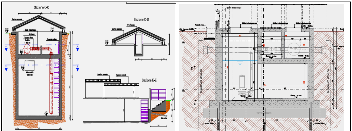
Sezione del progetto precedente con tetto a falde sporgete sul piano di campagna
