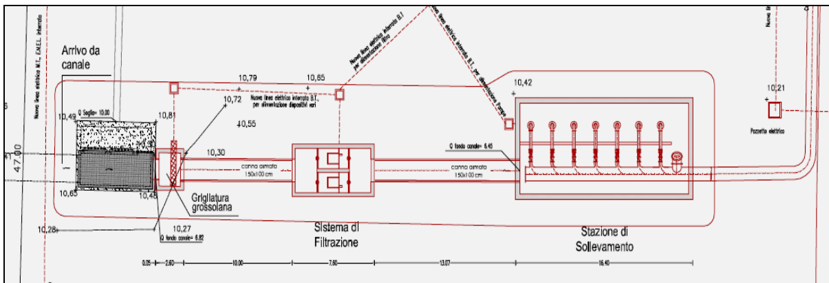
Planimetria della stazione di sollevamento nella condizione del precedente progetto
