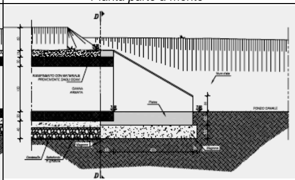
Sezione a monte
